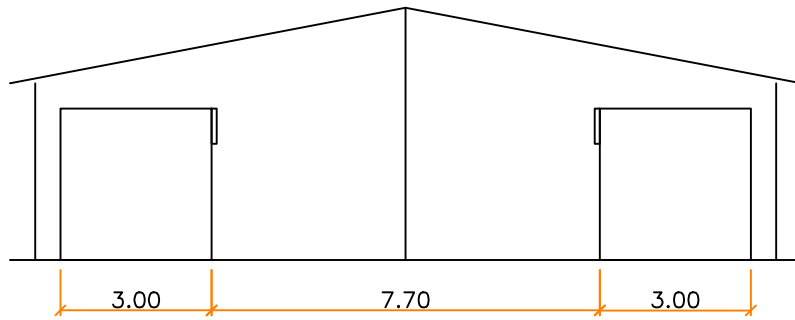
CORTE B-B': ESTANDES esc 1:200
