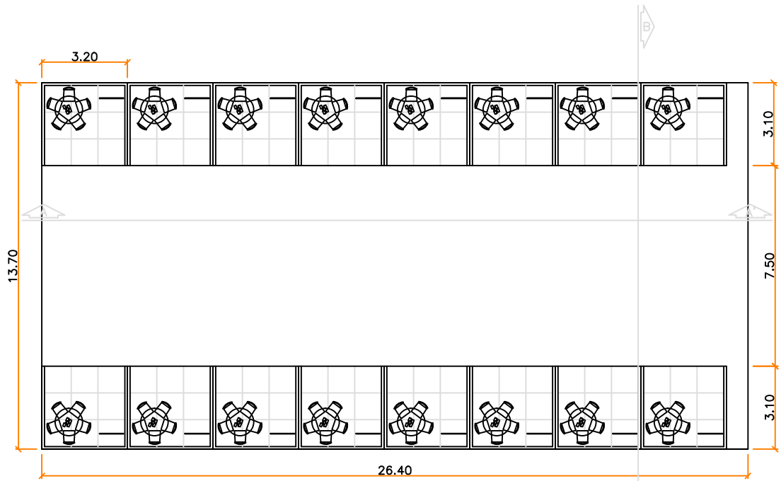
PLANTA BAIXA: ESTANDES esc 1:200
